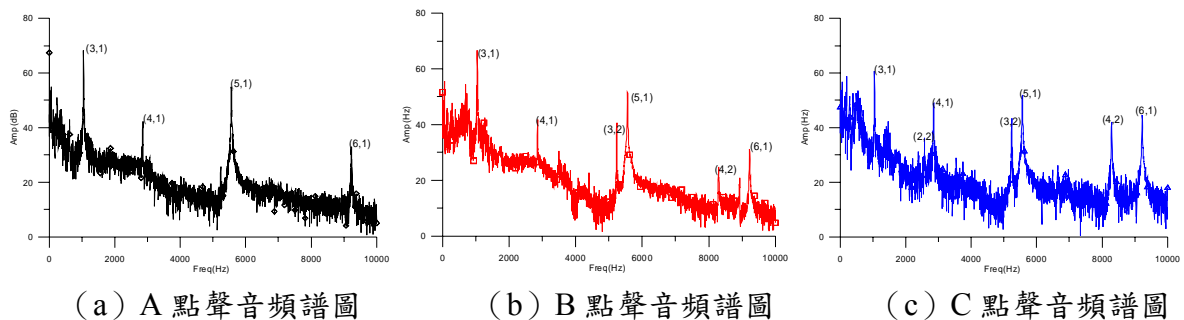
圖 10、不同位置之聲音頻譜圖
